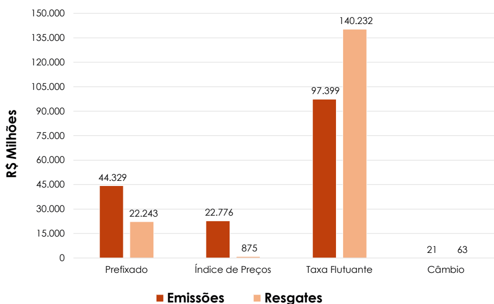
Gráfico 1.1 Emissões e resgates da DPMFi, por indexador Março/2021
