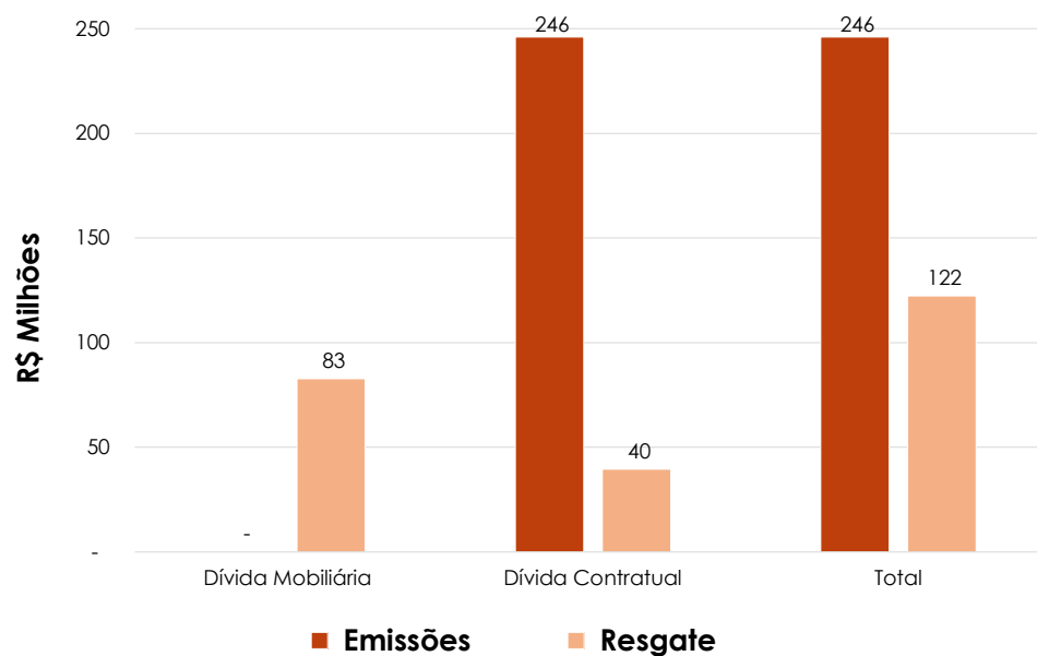
Gráfico 1.2 Emissões e resgates da DPFe Março/2021
