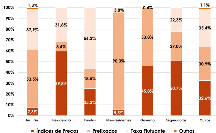
Gráfico 2.2 Composição da carteira de títulos públicos por indexador, por detentor—DPMFI Março/2021
