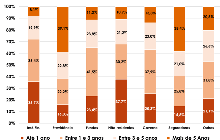
Gráfico 2.3 Distribuição por prazo de vencimento, por detentor—DPMFI Março/2021
